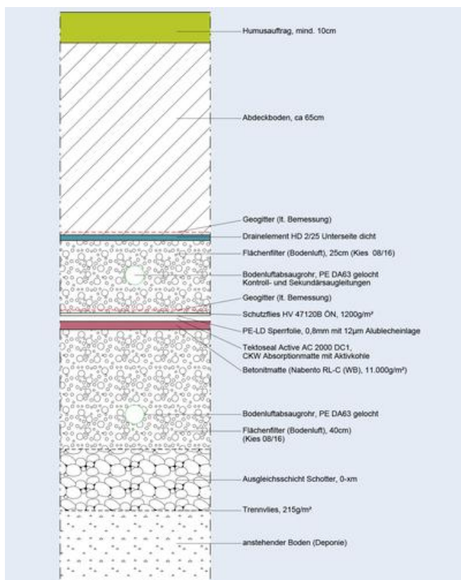
Aufbau der multifunktionalen Oberflächenabdichtung Bild: IAT GmbH
