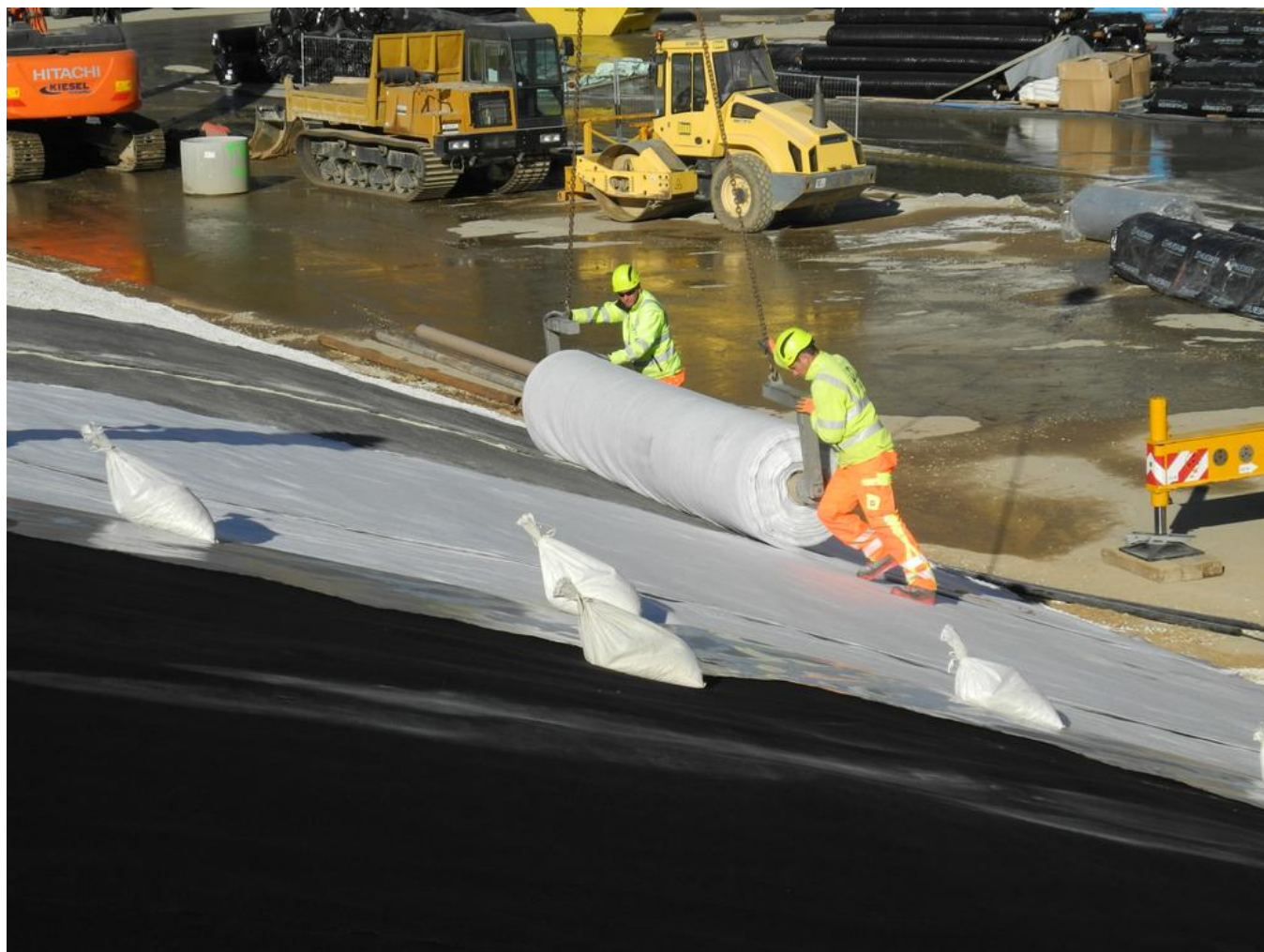
Verlegung der Oberflächenabdeckung. Bild: IAT GmbH
